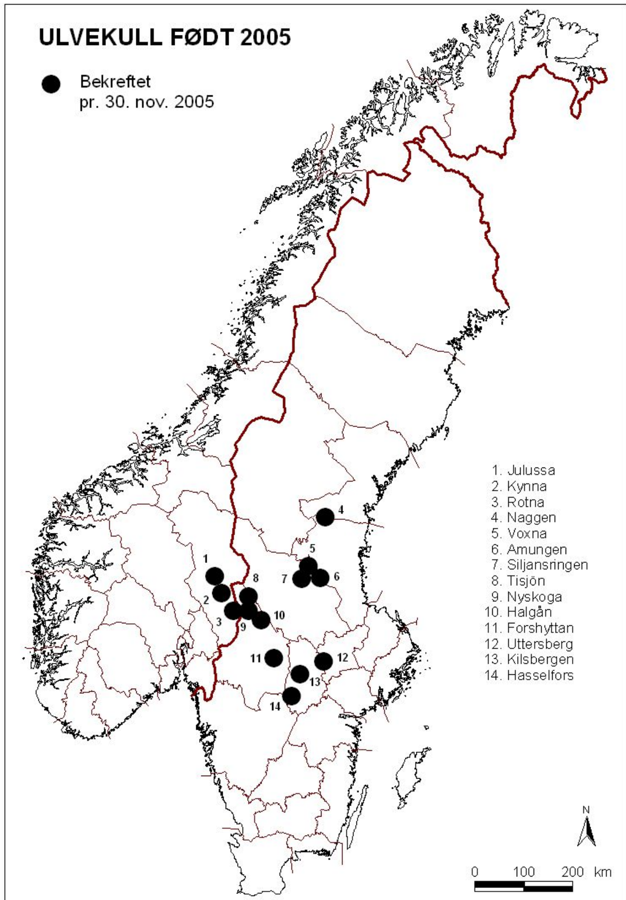
Figur 1. Foreløpig utbredelse av ulvereproduksjon i Norge og Sverige, hittil bekreftet i 2005 (oversikt pr. 30. november).
